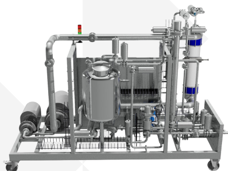
Установка BMF-18 Compact S1 – производительность 3-6 гл/час
